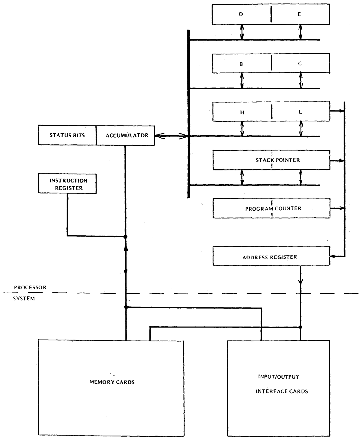
8080 PROCESSOR FIG. 1
